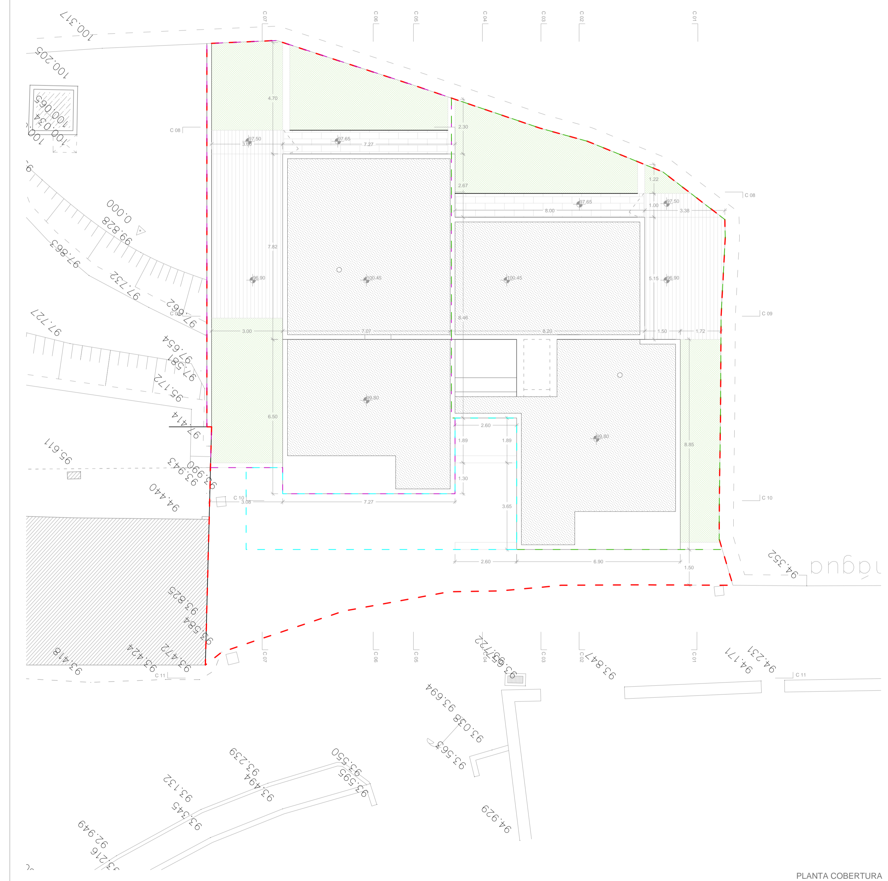
PLANTA COBERTURA
